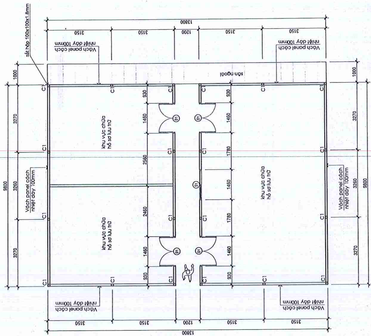
MẶT BẰNG KHO LƯU TRỮ TL: 1/70
