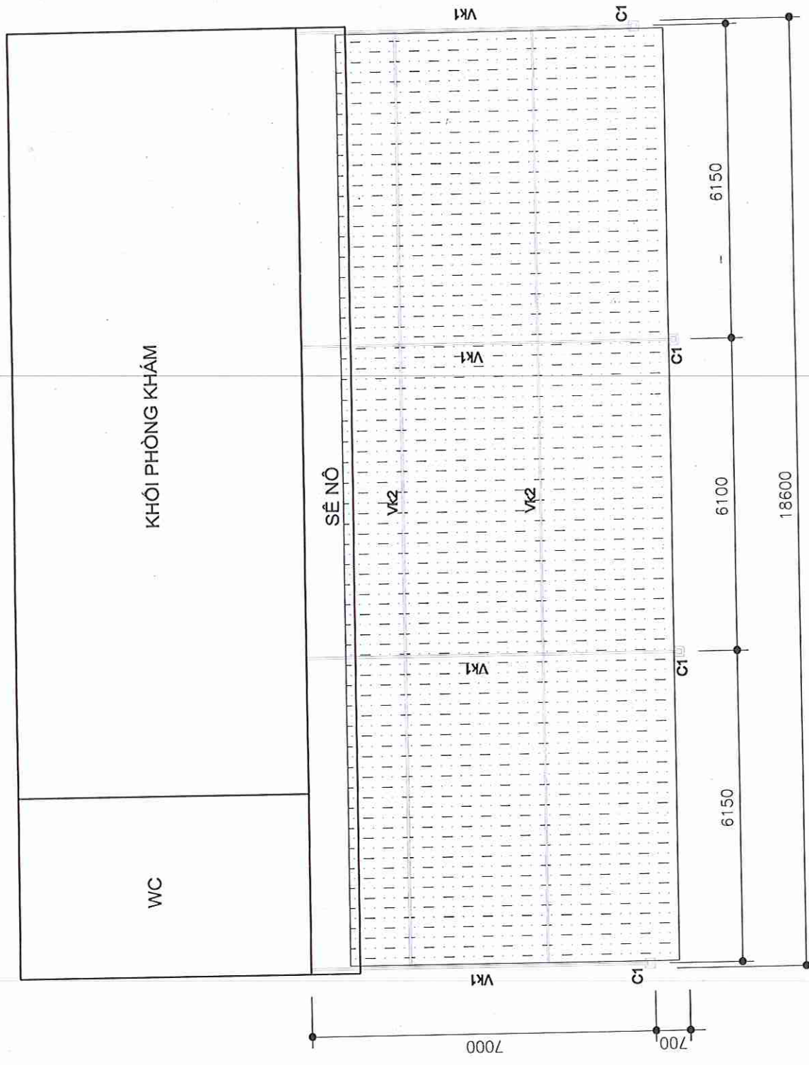
MẶT BẰNG HIỆN TRẠNG MÁI CHE KHU KHÁM BỆNH
