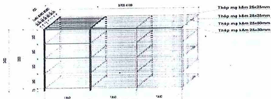
CHI TIẾT KỆ HỒ SƠ - SL: 02 CÁI
